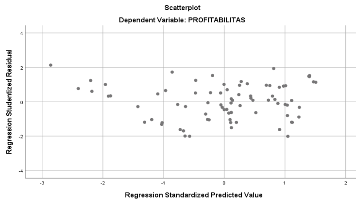
Gambar 2. Uj Heteroskedastisitas
